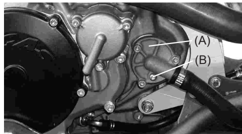
(A). Tapa bomba agua. (B). Tapón vaciado líquido refrigerante.
