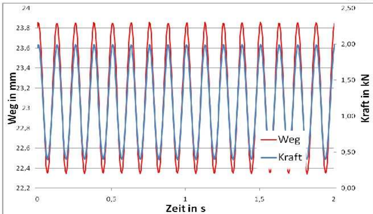
Diagramm 1: Kraft- und Wegverlauf Prüfung Stufe 1
