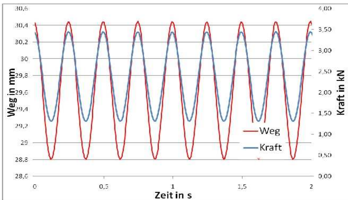
Diagramm 2: Kraft- und Wegverlauf während Prüfung Stufe 2
